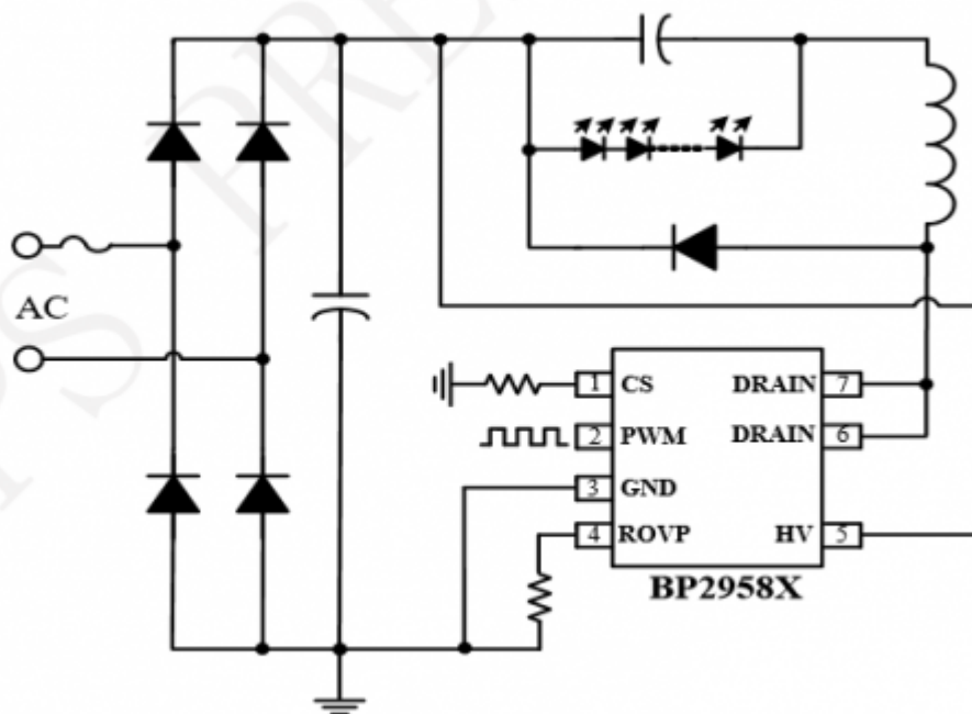
图 1 BP2958X 典型应用图
