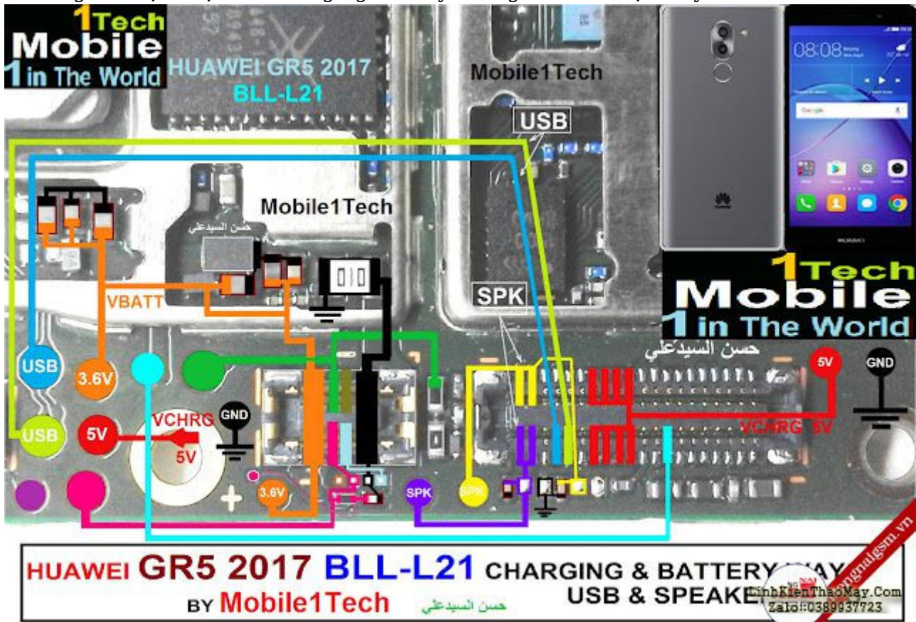
Sơ đồ sửa chữa điện thoại HUAWEI GR5 2017
