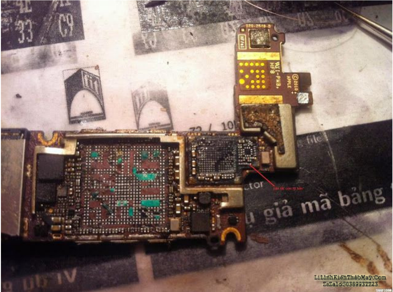
Tháo siêu ic wifi iphone 4 và cấu tắt tụ như hình sau
