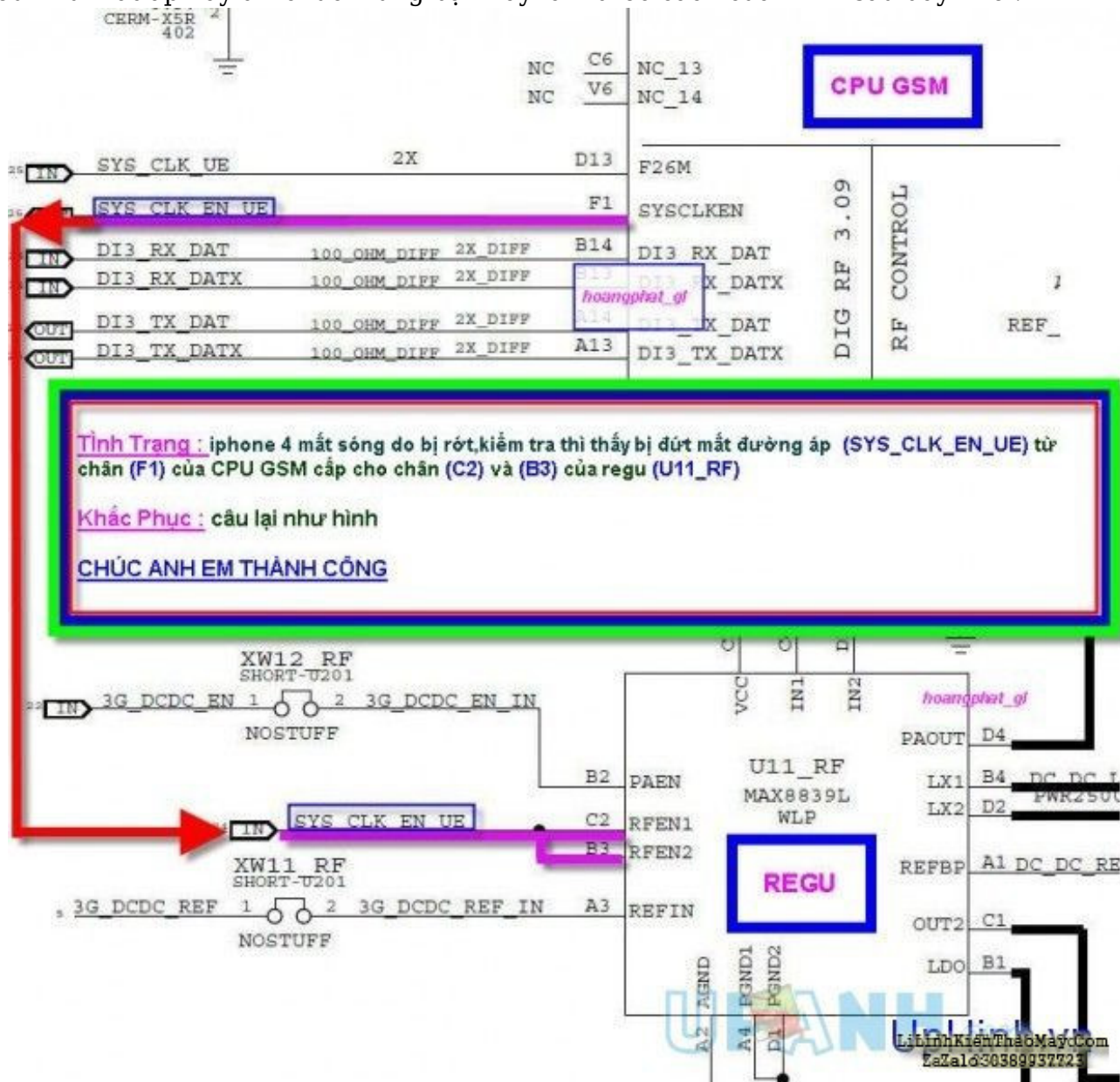
Sơ đồ câu áp SYS_CLK_EN_UE
