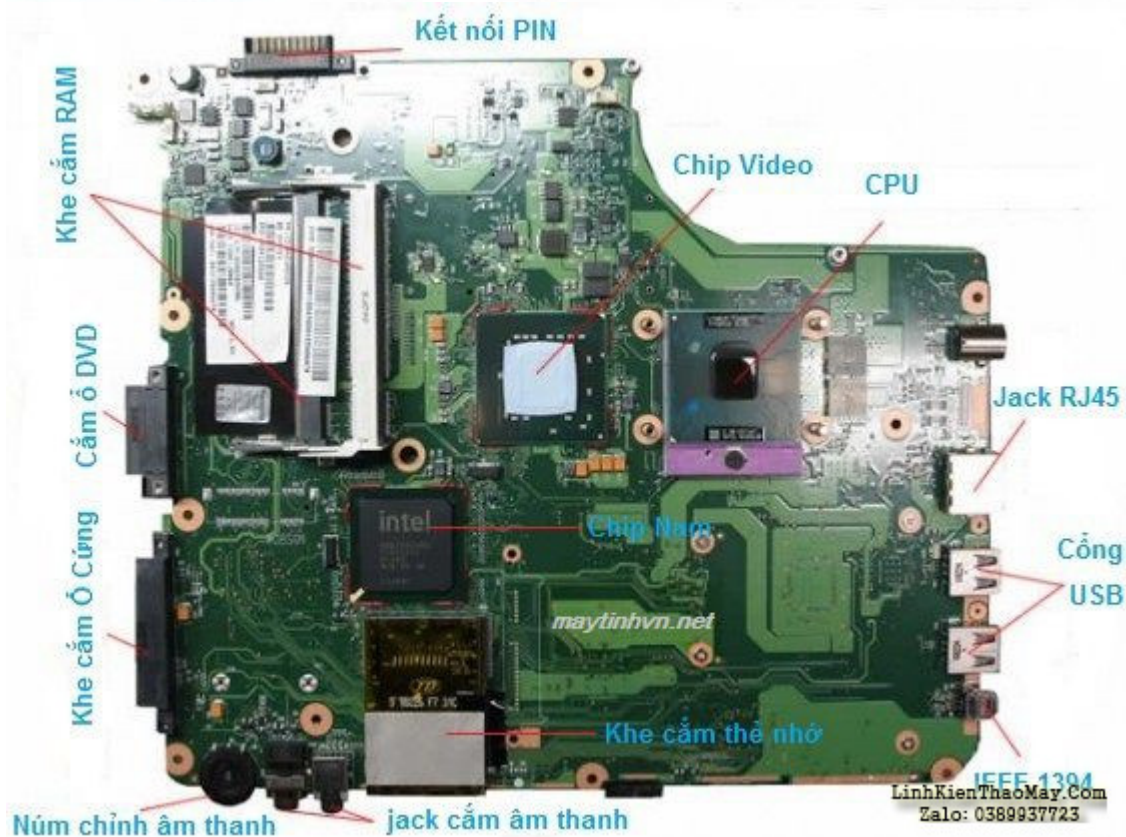
Các linh kiện trên mainboard Laptop
